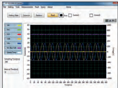
Aufzeichnung der einzelnen Parameter wie Spannung und Strom der einzelnen Phasen.
